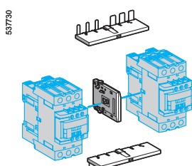
LAD 9R3
