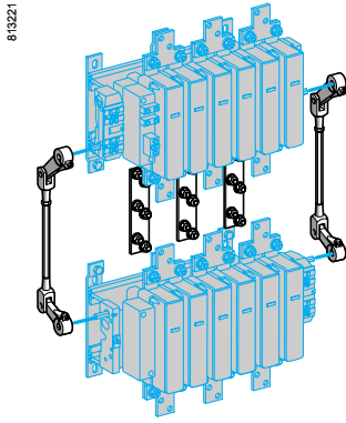
LA9 FX970
